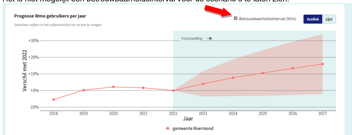
Figuur 12: Betrouwbaarheidsinterval
